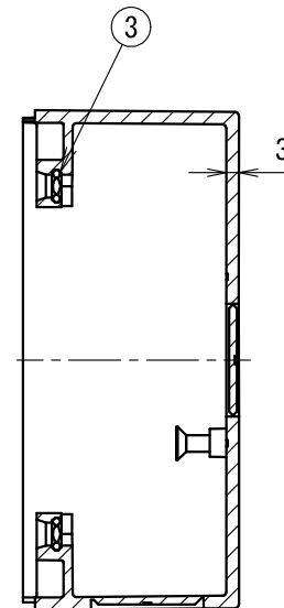
断面 A-A
